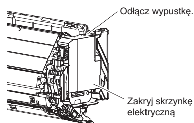
Rysunek 1: Zdejmij pokrywę ze skrzynki elektrycznej
