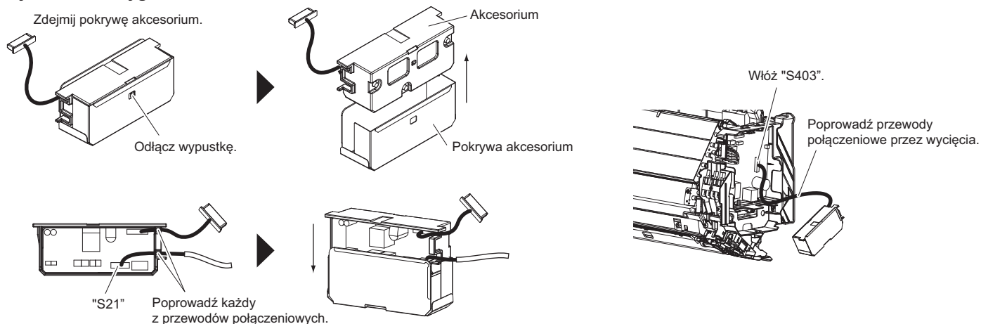
Rysunek 2: Przygotowanie akcesorium
