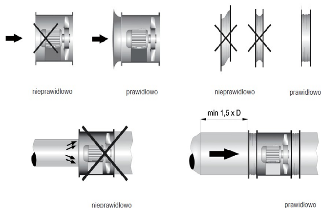
PRZYKŁAD MONTAŻU WENTYLATORÓW OSIOWYCH AXEL, AXEL.L
