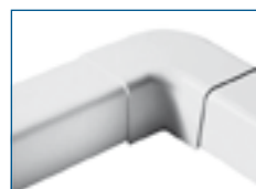
kąt płaski
