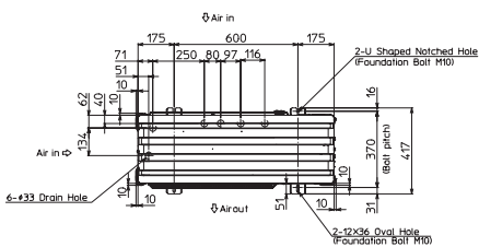
MXZ-4E83VAHZ
