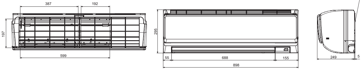
Urządzenia ściennie PKA-RP35/50 HAL
