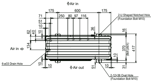
MXZ-6D122VA
