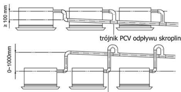
sposób podłączenia kilku jedn. wewnętrznych do odpływu skroplin
