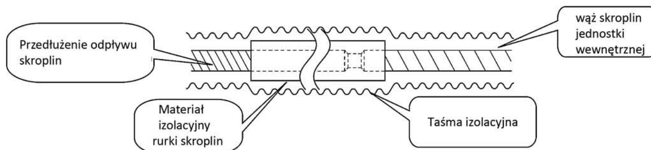
Schemat podłączenia węża skroplin jednostki wewnętrznej z rurą odpływu skroplin
