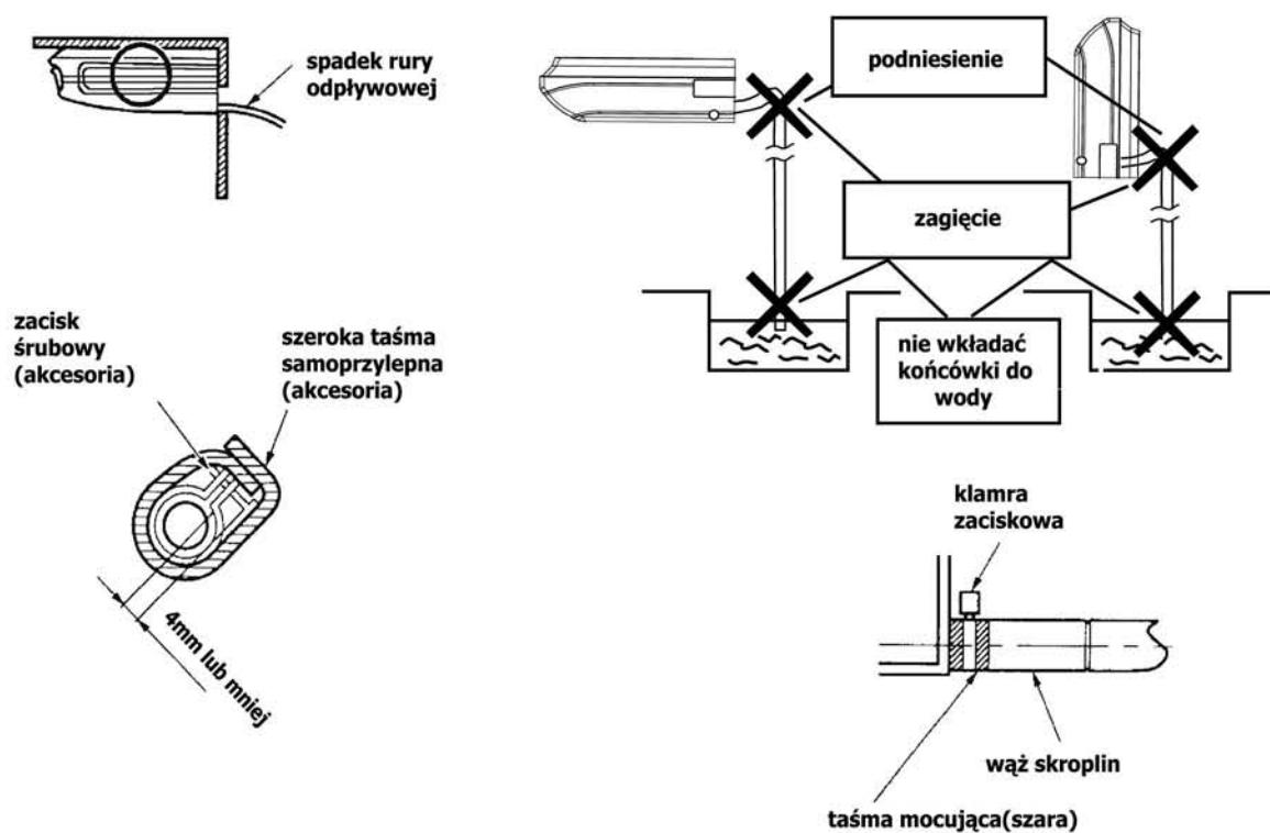
Schemat podłączenia węża skroplin jednostki wewnętrznej z rurą odpływu skroplin
