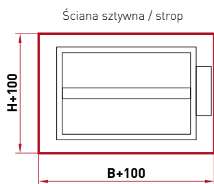
Rysunek 3. Wymagane otwory dla kłapy KWP-O montowanej pojedynczo.
