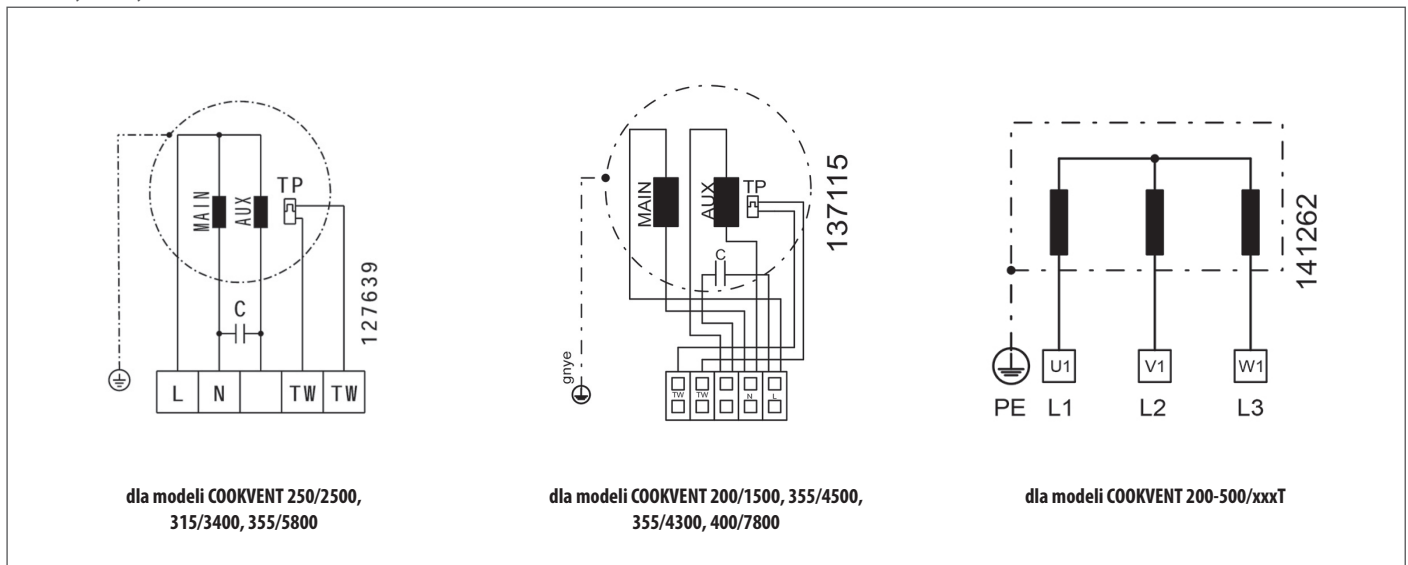
schematy elektryczne
